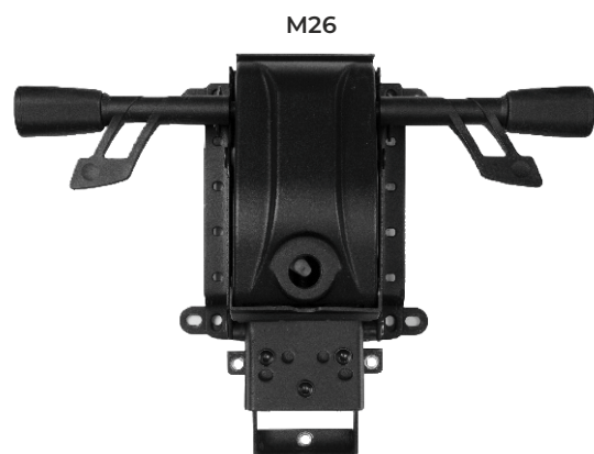
Синхромеханизм качения MULTIBLOCK
